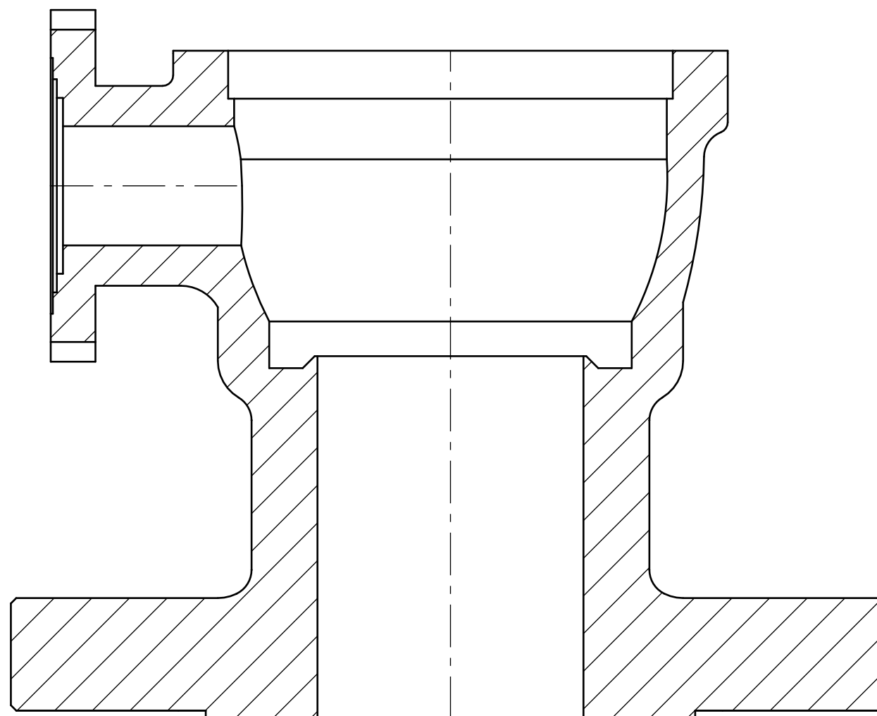
SEZIONE A-A SCALA 1:1
